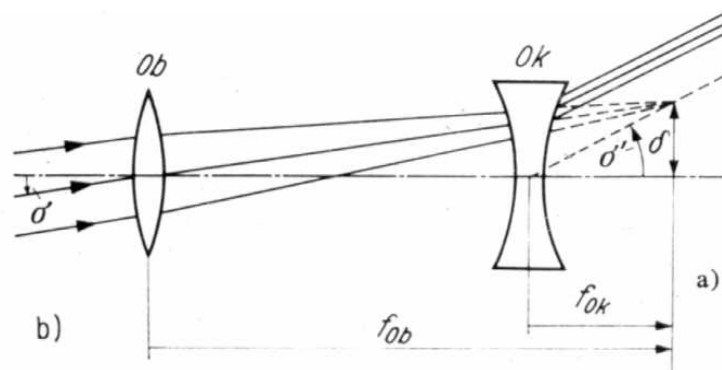
Abb. 9 Strahlengang im Galilei Fernrohr Quelle: MARTIN-LUTHER-UNIVERSITÄT HALLE-WITTENBERG, INSTITUT FÜR PHYSIK, FG FESTKÖRPERANALYTIK
